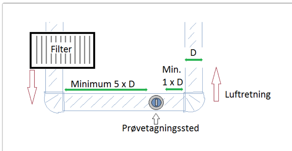
Figur 1. Prøvetagningssted skal etableres, så turbulens minimeres.
