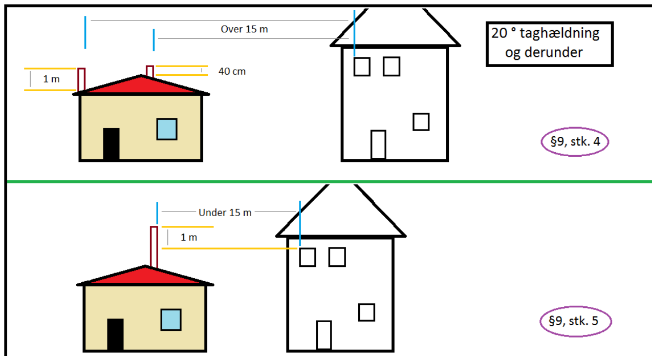
Figur 2. Minimumshøjder på afkast (skorsten) afhængigt af øvre kant på døre, vinduer og luftindtag. For taghældning 20° og derunder i relation til §9, stk. 4, punkt 1 samt §9, stk. 5.
