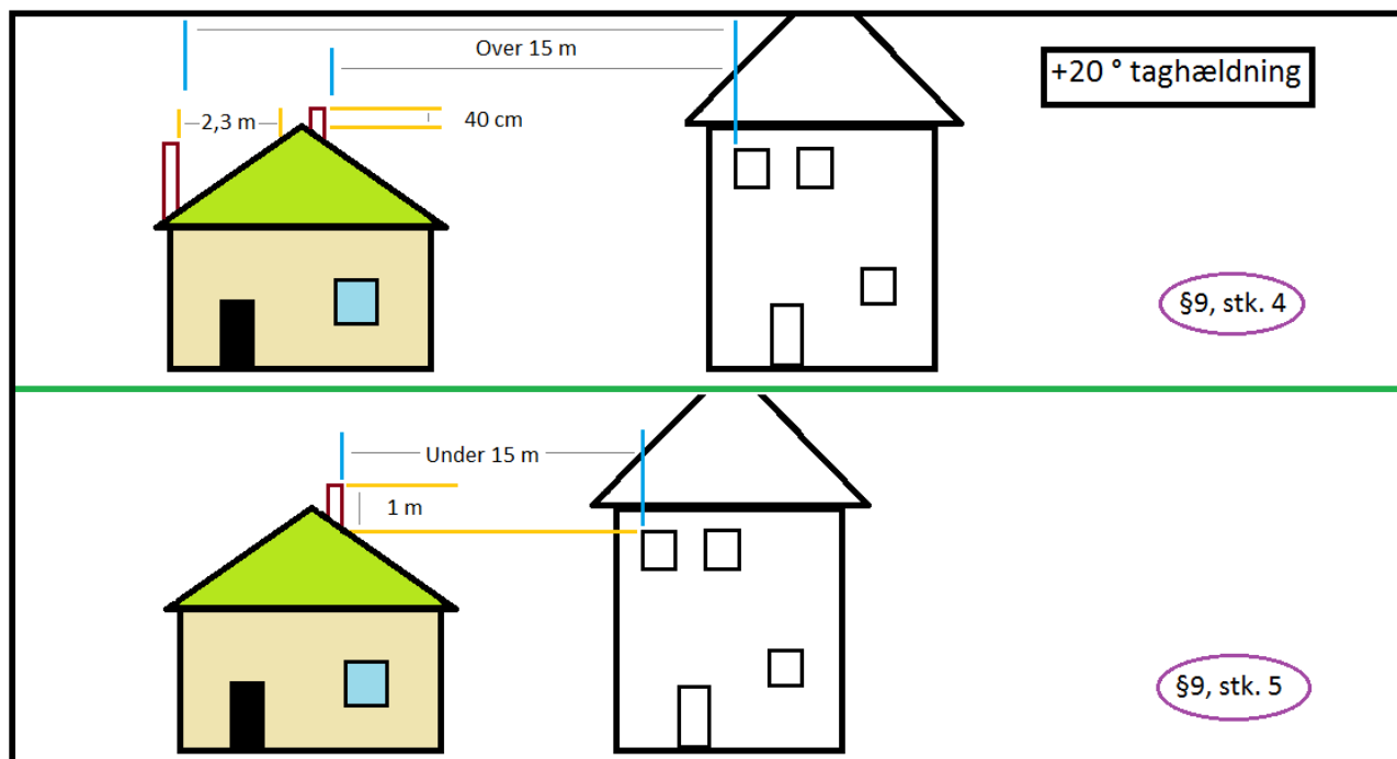
Figur 3. Minimumshøjder på afkast (skorsten) afhængigt af øvre kant på døre, vinduer og luftindtag. For taghældning over 20° i relation til §9, stk. 4, punkt 2 samt §9, stk. 5.
