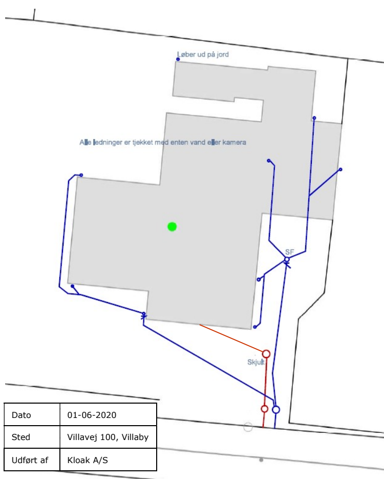
Billede 1 Eksempel på kloaktegning
