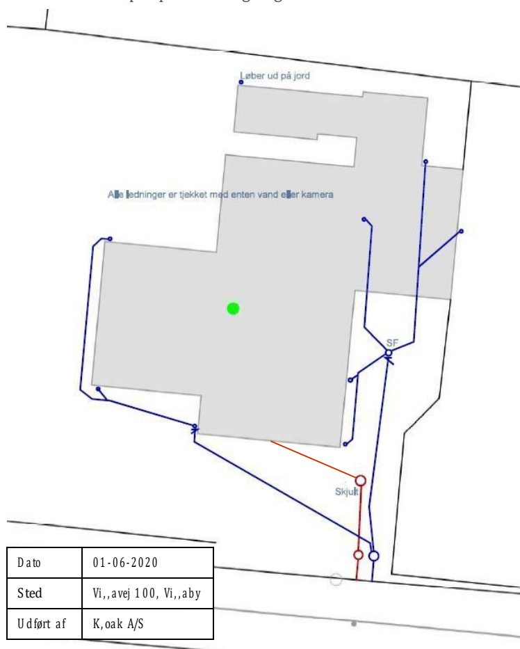
Billede 1 Eksempel p& kloaktegning
