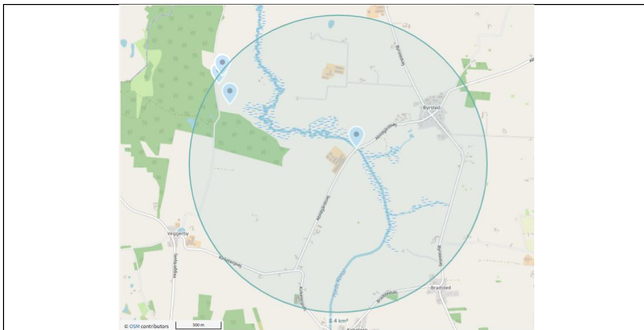
Resultat af søgningen på fund af bilag IV-arter i en radius af ca. 1,5 km fra staldanlægget (kort fra arter.dk, openstreetmap.org/copyright). Søgning foretaget d. 12/8-2025.
