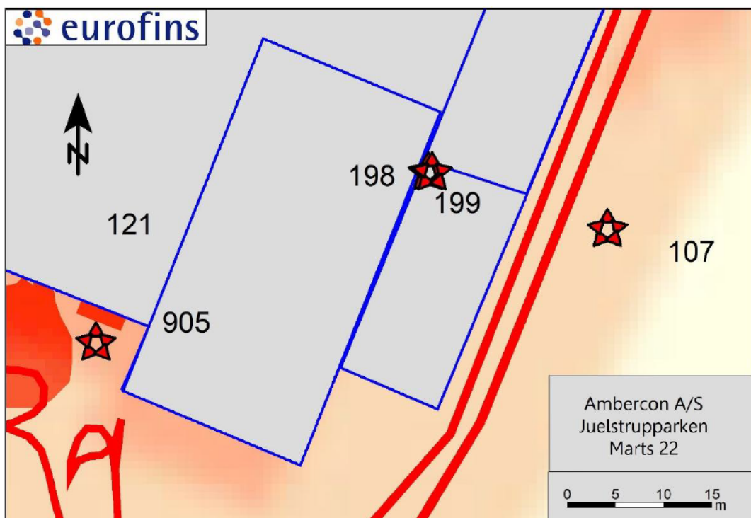
Figur 2. Støjkilde 198 og 199 er ventilationsanlægget og afkastet. Begge er sat ind i beregningen med en kildestyrke på 78 dB(A).
