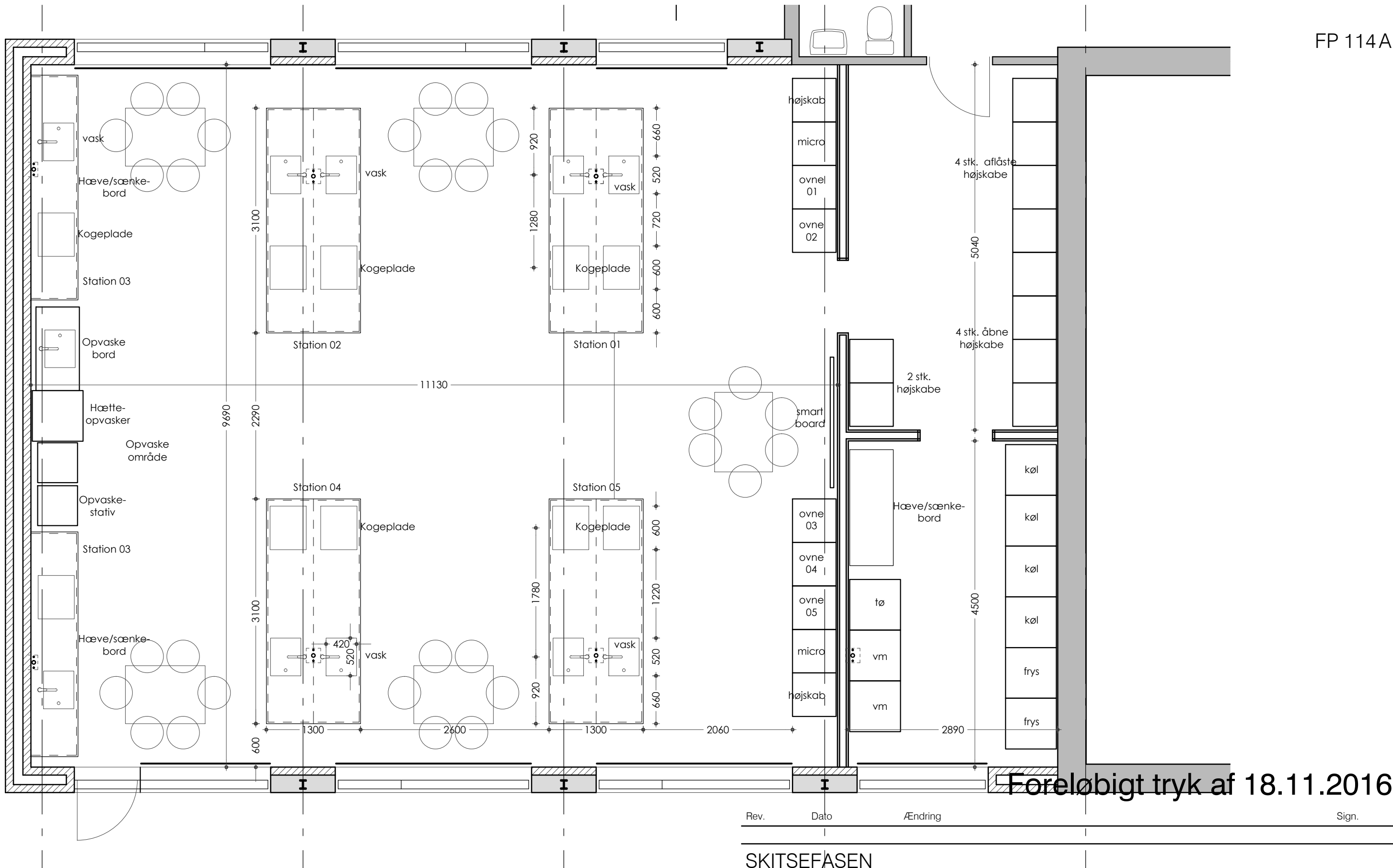
PLAN 1:50
