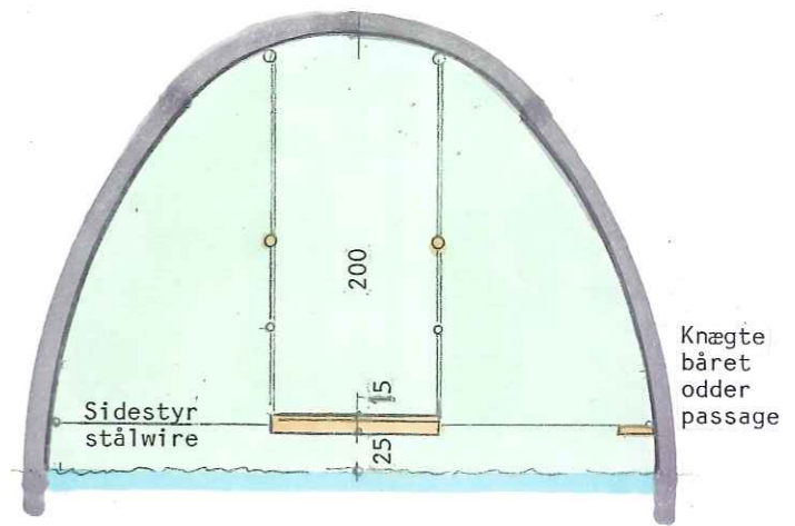
TVÆRSNIT
