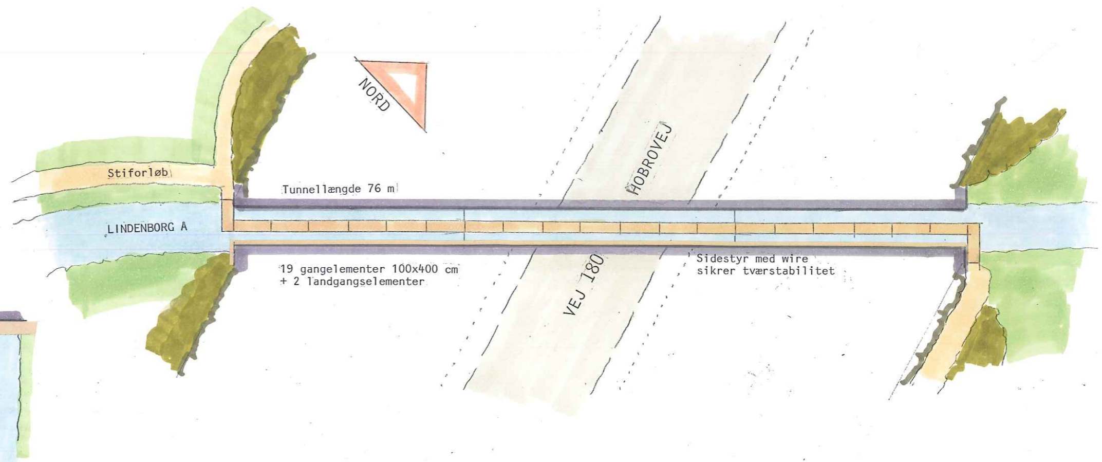
OVERSIGTSPLAN 1:400
